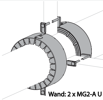
Wand: 2 x MG2-A U
