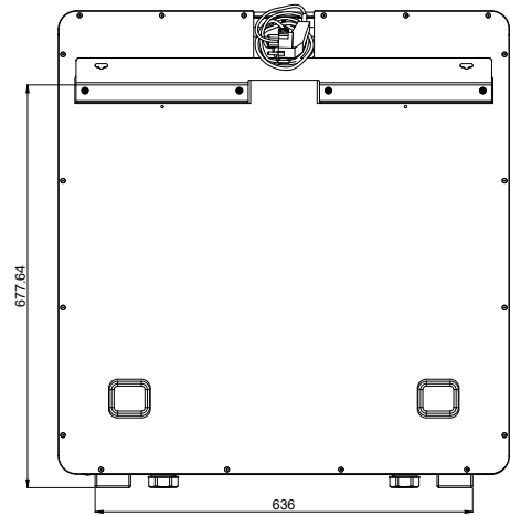
Achteraanzicht
