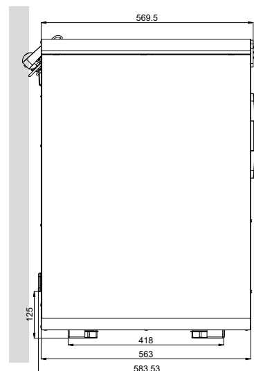
Zij-aanzicht
