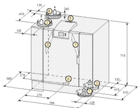
Rechter-uitvoering 2/2
