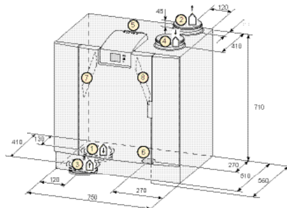
Linker-uitvoering 2/2
