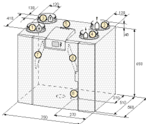
Linker-uitvoering 4/0
