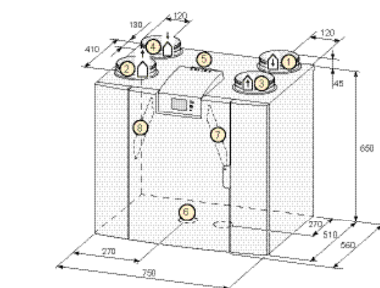
Rechter-uitvoering 4/0
