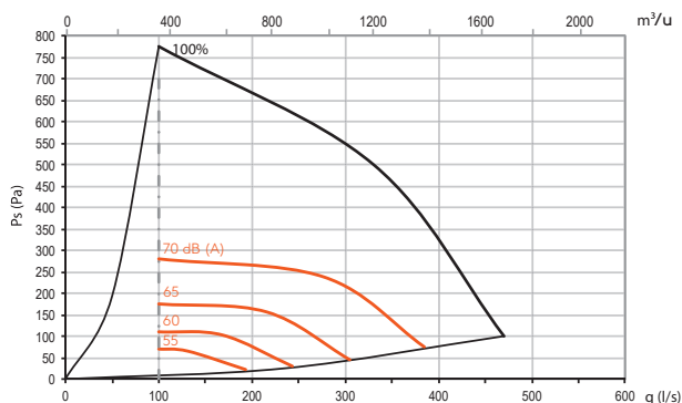
Geluidsvermogen niveau naar het pulsiekanaal / afblaaskanaal
